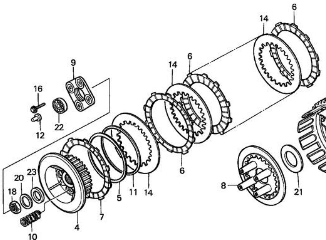
Schemat: Honda XL600V Transalp PD10
